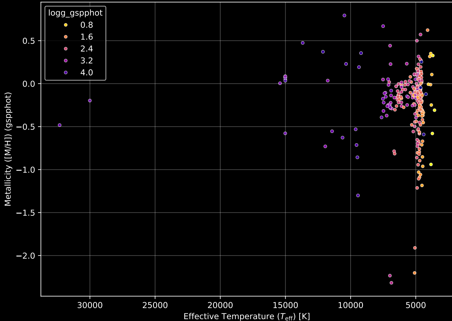
APOGEE DR17 Field: [154+00] Stellar Population Parameters (n= 274)
